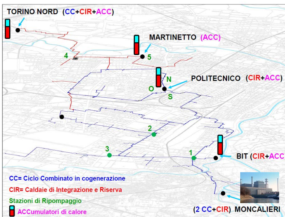
Impianti di produzione e accumuli rete di teleriscaldamento di Torino.
