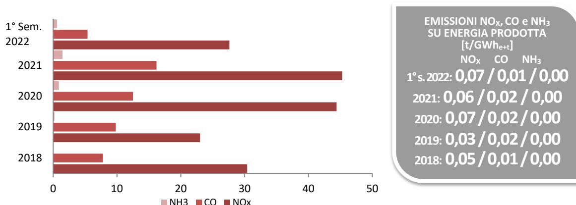
Grafico 4: Emissioni in atm. NO x - CO - NH 3 da combustione CCGT e Caldaie [t]
