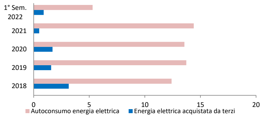
Grafico 3: Consumo di energia elettrica [GWh]
