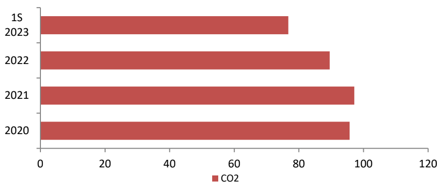
Grafico 4: Emissioni in atmosfera CO 2 [t] da GE e caldaie riscaldamento
