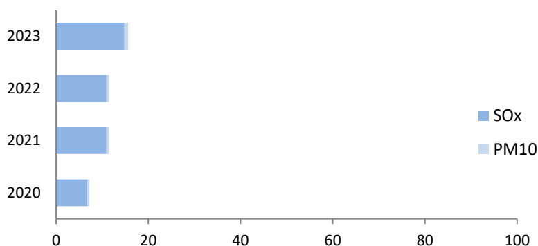
Grafico 6: Emissioni in atmosfera evitate di SO x e PM10 [t]
